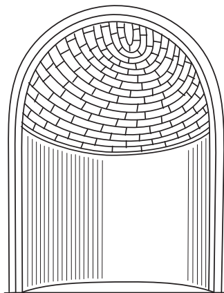
Voûte en cul-de-four
